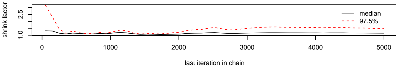
beta0[4]
