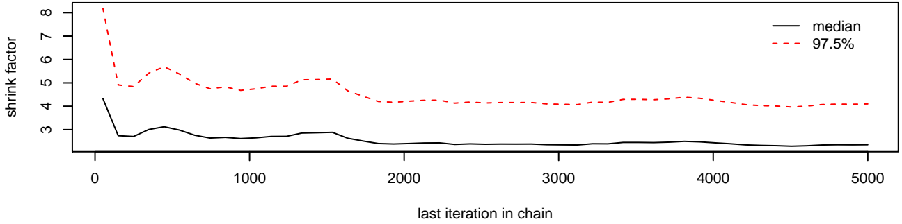
alpha0[2]
